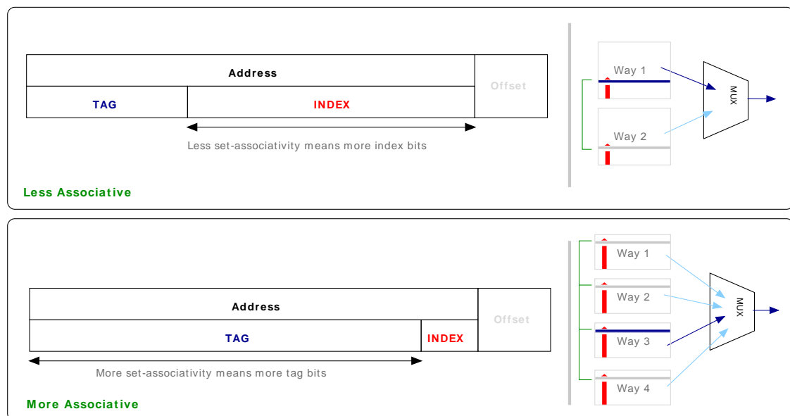
Figure 3.5. Cache tags
